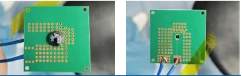
△ RTO 加载透镜实物
